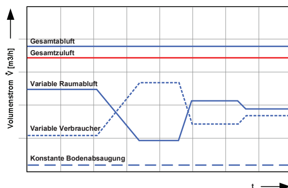
Bild 1: Variable Raumabluft
